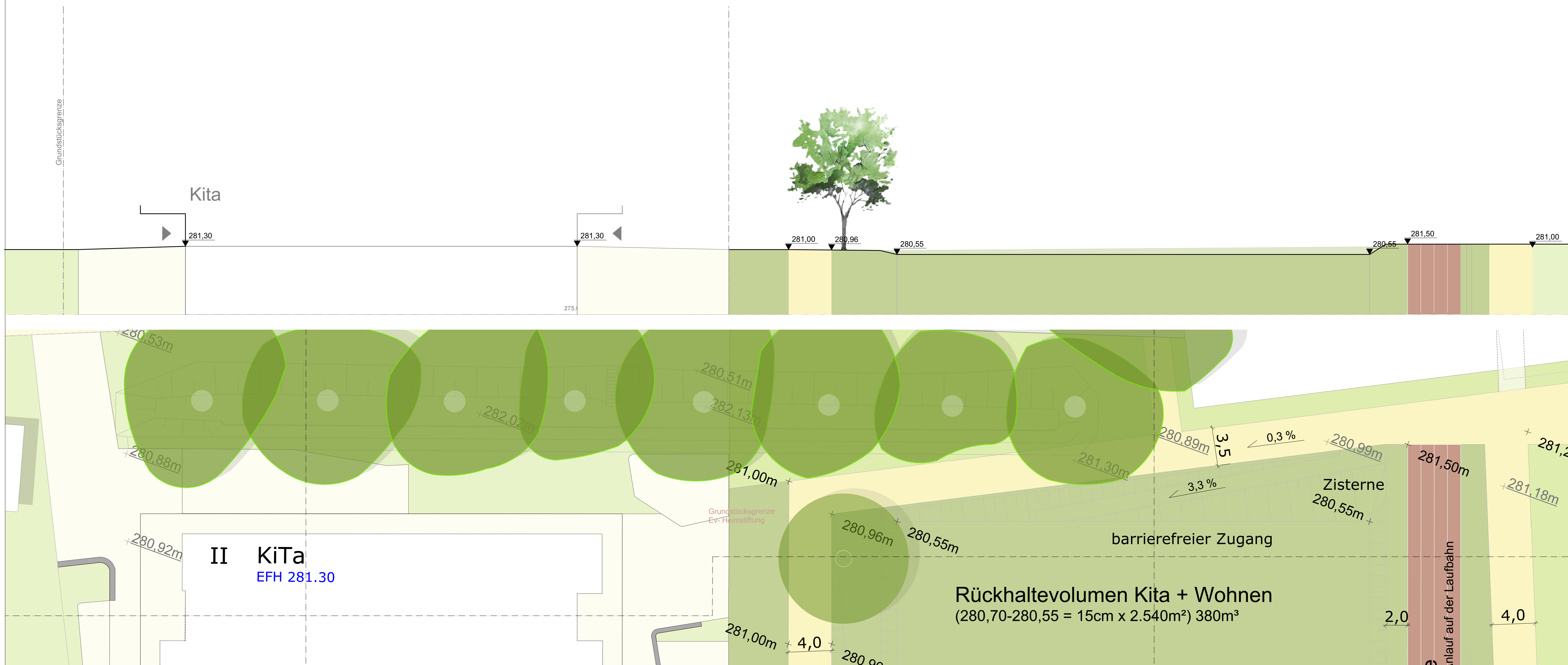
Schnitt A-A M 1:200
