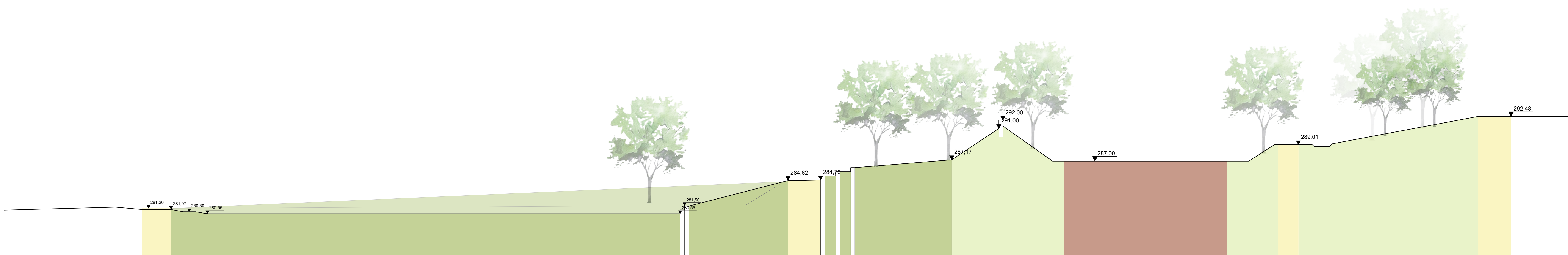
Schnitt B-B M 1:200
