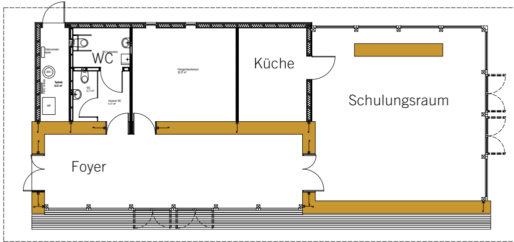
Grundriss
